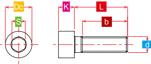
CAP BOLT M6 P=1.0 L 10 mm – 45 mm
